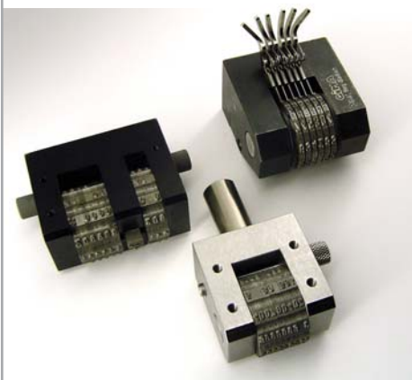
Maschinenprägwerke
